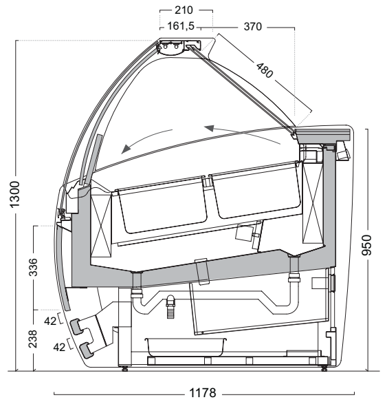
Dimensiones perfil P60 con panel frontal
