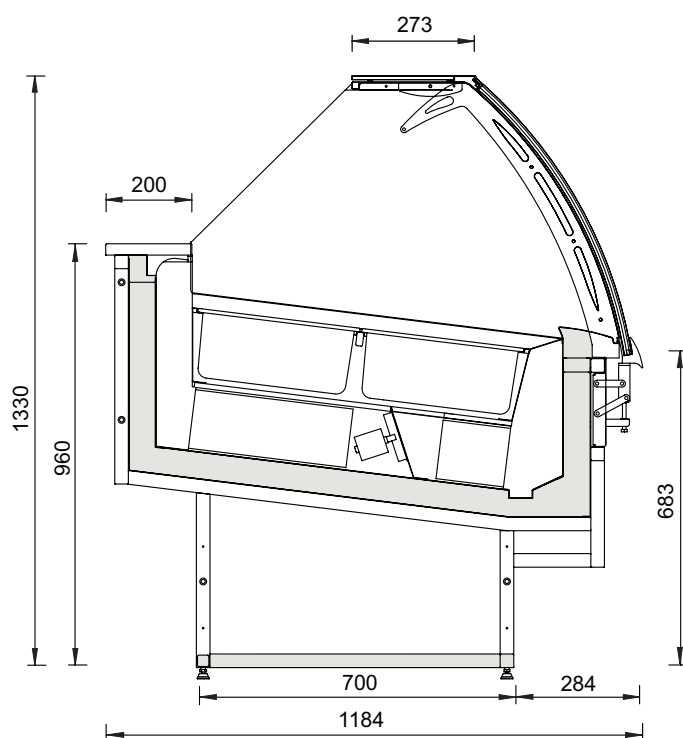
Dimensiones perfil Matrix heladería
