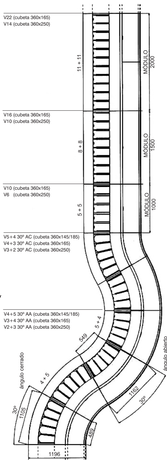
Diferentes posibilidades de cubeta en Matrix curva
