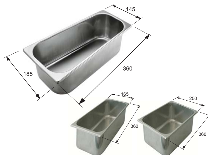
Diferentes posibilidades de cubeta en Matrix curva
